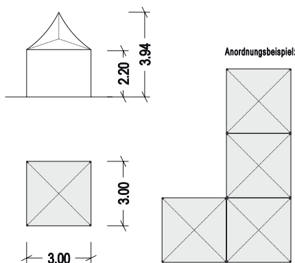
Grundriss 3 x 3 m
