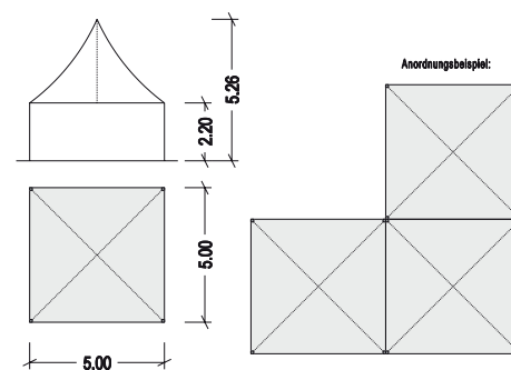
Grundriss 5 x 5 m
